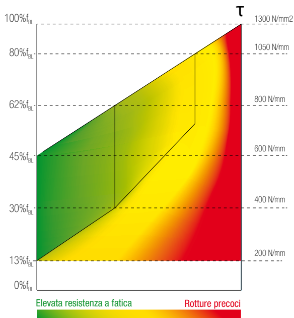
FIG.2 Condizioni di Lavoro e Resistenza a Fatica
